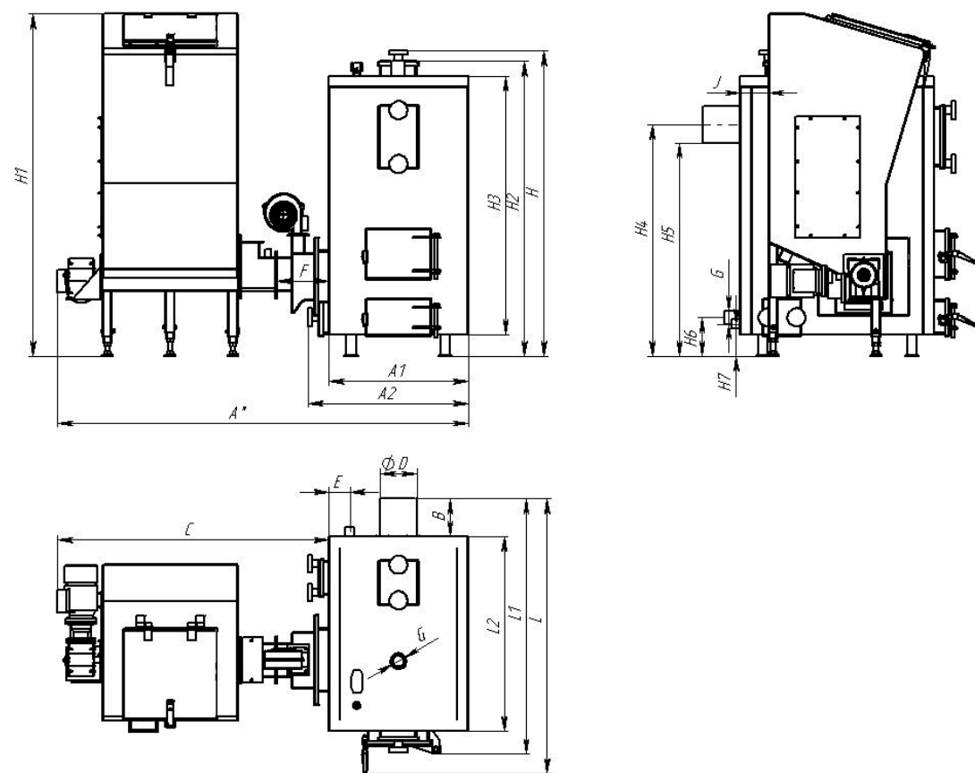
Рис. 6 Котел с боковым бункером (АПТ)
