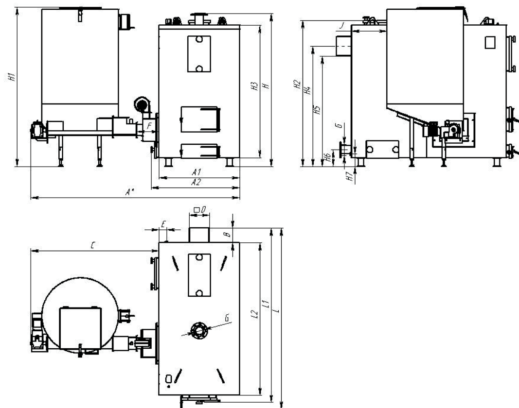
Рис. 9 Котел с передним бункером (АПТ)
