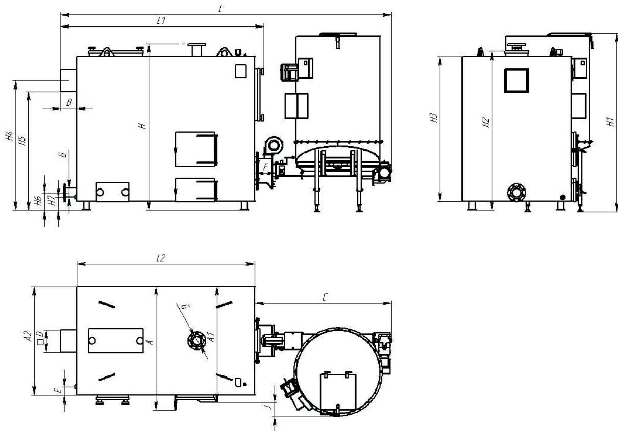
Рис. 7 Котел с боковым бункером (АПТ)
