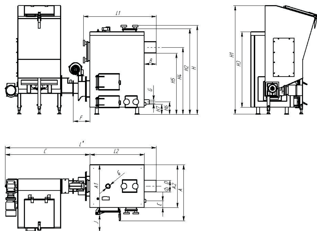
Рис. 8 Котел с передним бункером (АПТ)
